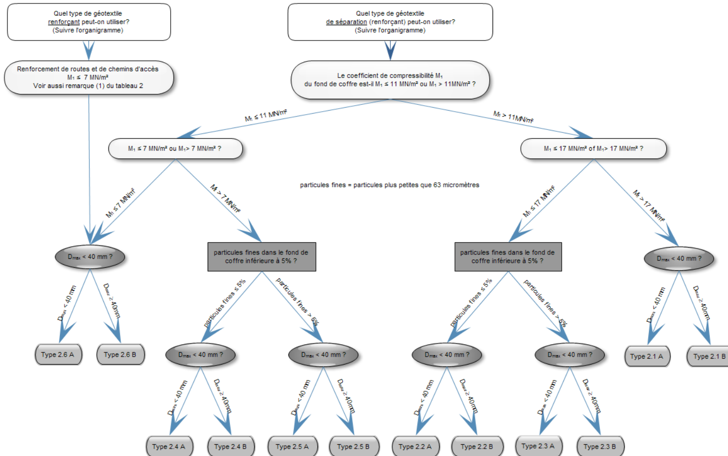
Figure 1 – Organigramme pour la détermination du type de géotextile
